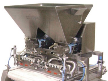
Dépoteurs de fondant à moteurs servos
